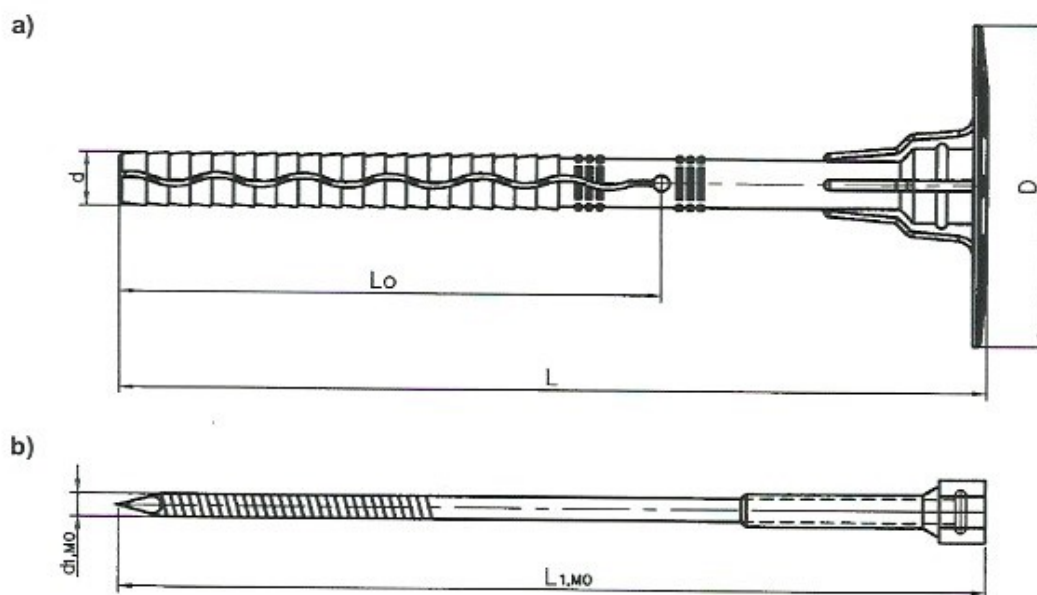
Rysunek A7. Łącznik tworzywowo-metalowy ŁIM do mocowania termoizolacji a) tuleja tworzywowa, b) trzcień stalowy z główką pokrytą powłoką tworzywową
