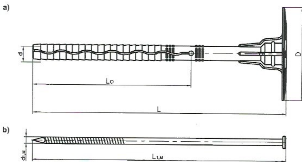
Rysunek A8. Łącznik tworzywowo-metalowy ŁIM-S do mocowania termoizolacji a) tuleja tworzywowa, b) trzcień stalowy z główką niepokrytą powłoką tworzywową
