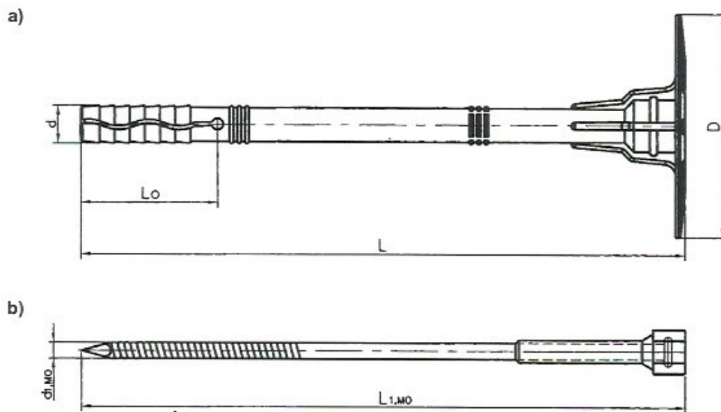
Rysunek A9. Łącznik tworzywowo-metalowy ŁIM-K do mocowania termoizolacji a) tuleja tworzywna, b) trzpień stalowy z główką pokrytą powłoką tworzywną
