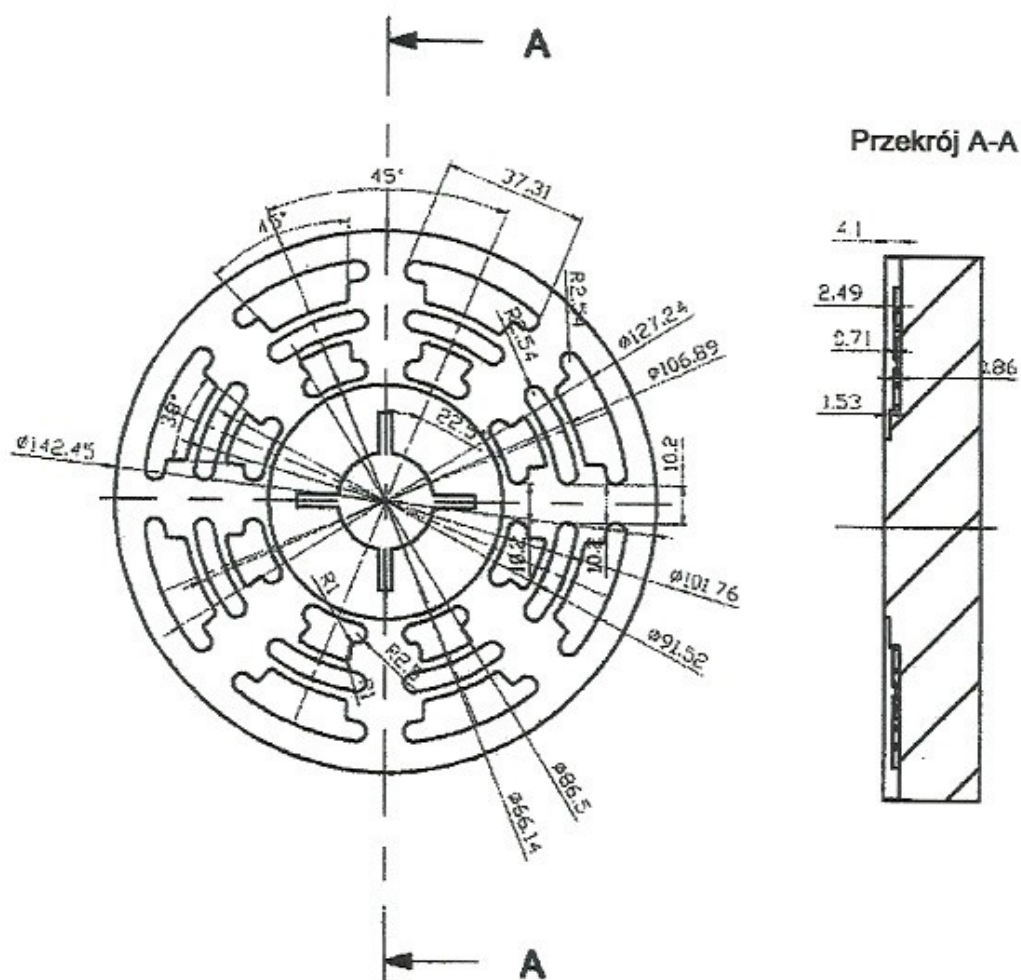
Rysunek A13. Dodatkowy, tworzywny talerzyk dociskowy TDW-140
