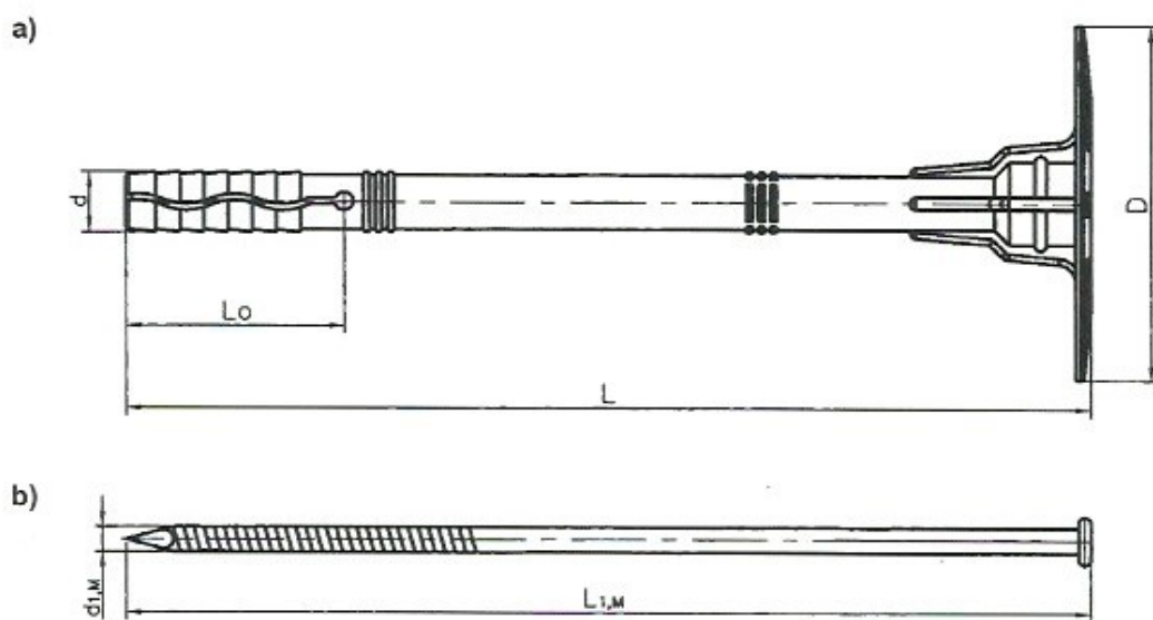
Rysunek A10. Łącznik tworzywowo-metalowy ŁIM-S-K do mocowania termoizolacji a) tuleja tworzywna, b) trzpień stalowy z główką niepokrytą powłoką tworzywną
