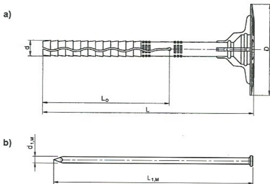
Rysunek A4. Łącznik tworzywo-metalowy ŁI-S do mocowania termoizolacji a) tuleja tworzywowa, b) trzcień stalowy z główką niepokrytą powłoką tworzywową
