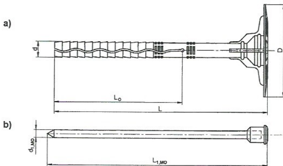
Rysunek A3. Łącznik tworzywo-metalowy ŁI do mocowania termoizolacji a) tuleja tworzywowa, b) trzcień stalowy z główką pokrytą powłoką tworzywową
